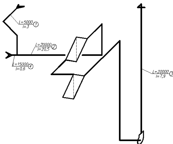
Рисунок 3. Схема аспирационной сети от дробильной установки.
