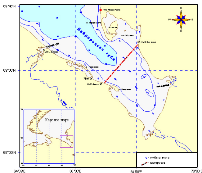
Рисунок – 1 Географическое положение Байдарачьей губы Карского моря и трасса перехода магистральных газопроводов
