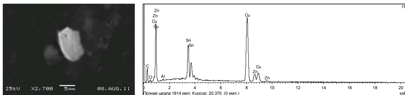
Рисунок - 1 Сплав Cu, Sn и Zn в пробе пыли, отобранной в зоне отчуждения МКАД (условия съёмки shadow, BSE) – а), и его энергодисперсионный спектр – б).
