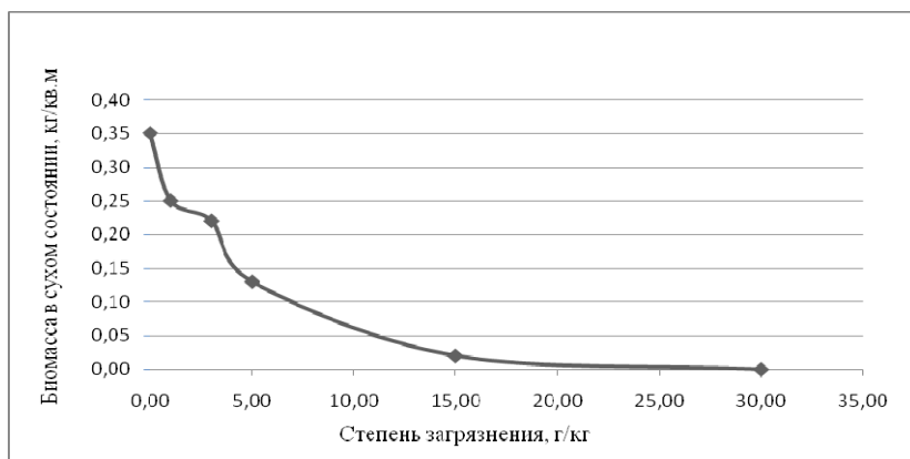
Рисунок 2 Зависимость биомассы растительности от степени загрязнения
