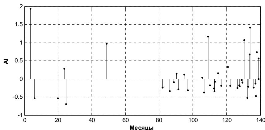
Рисунок 2. График наблюдённого альгоиндекса на акватории близ устья р. Песчанки
