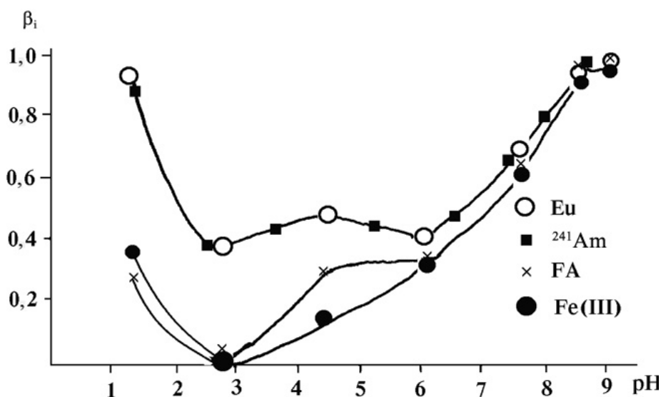
Рисунок - 1 Зависимость доли β растворенных форм 152 Eu, 241 Am, фульватной компоненты железофульвата и железа от рН
