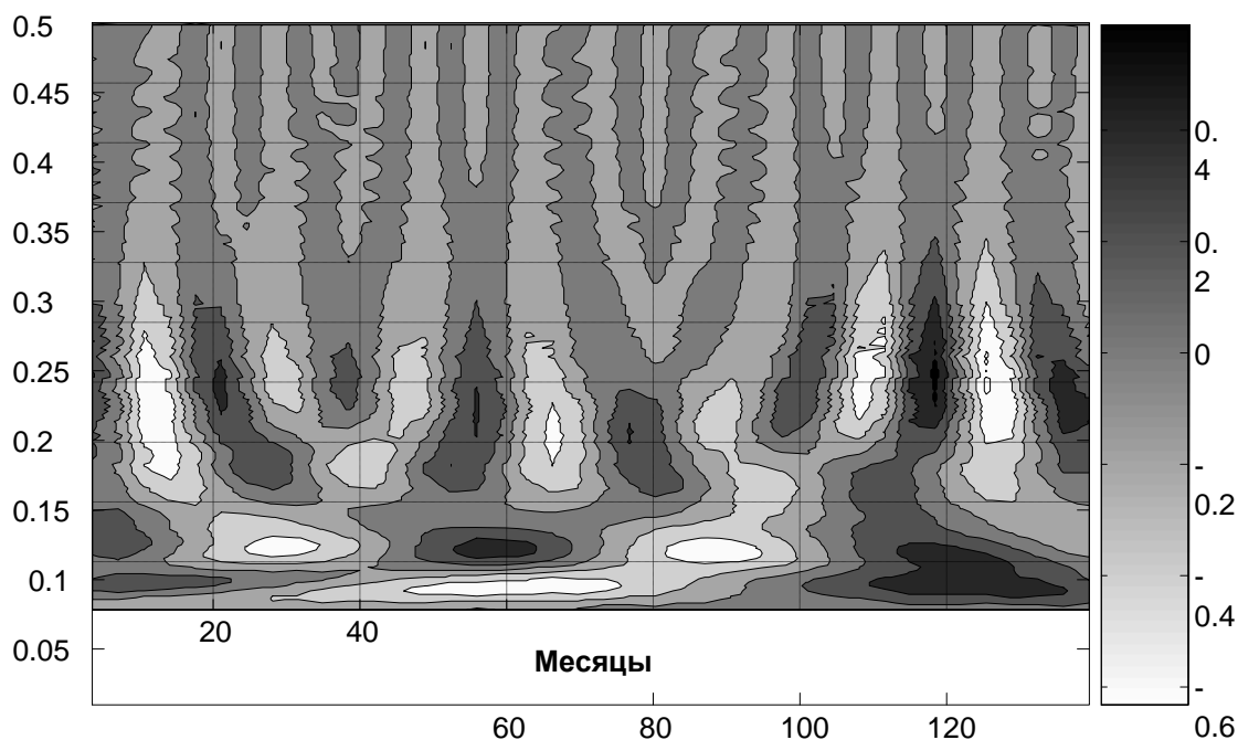
Рисунок 3. Вейвлетограмма изменения альгоиндекса.
