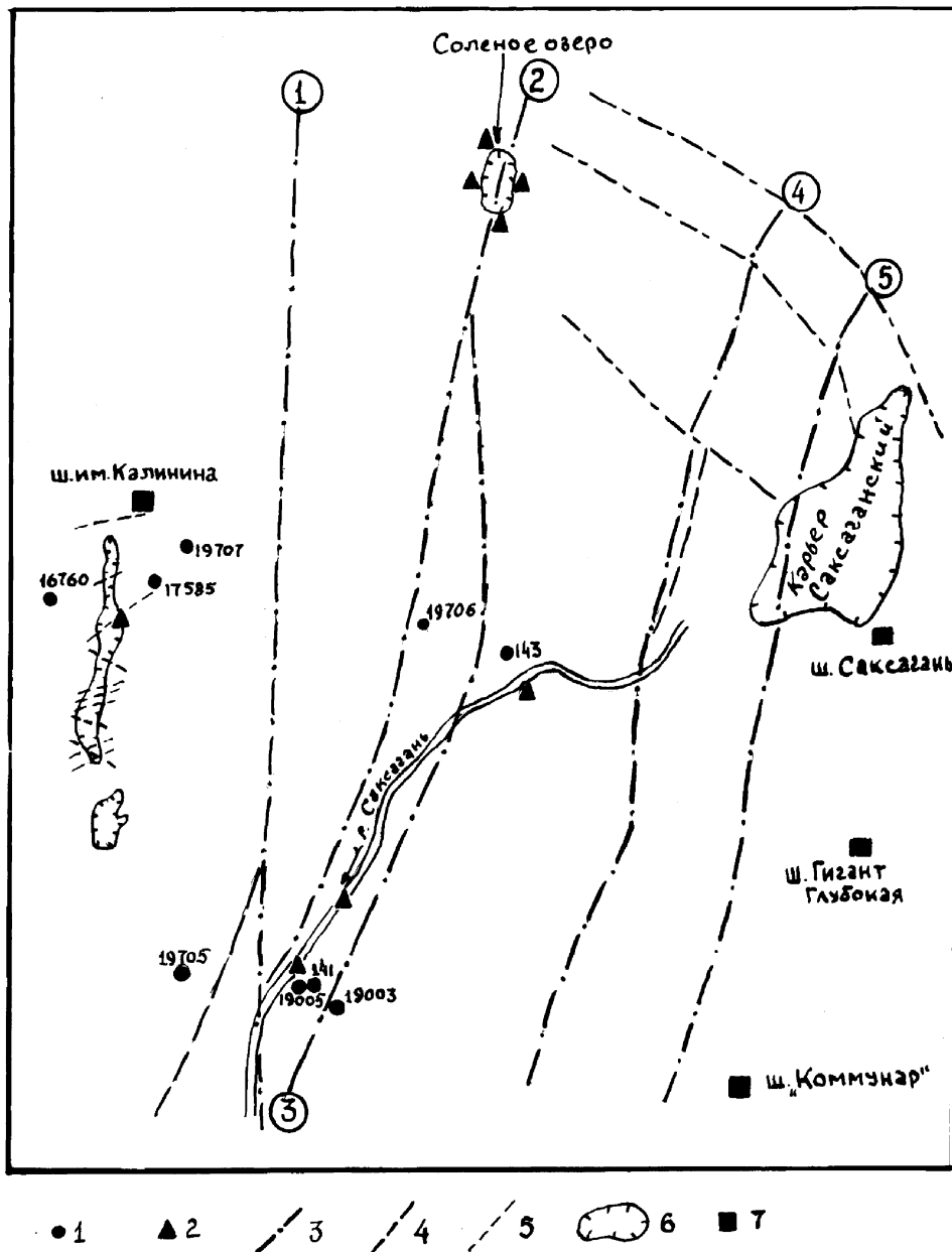
Рисунок 1 Схема района детальных исследований. Условные обозначения: пункты отбора подземных вод из скважин; пункты отбора поверхностных вод; основные разломы глубинного Криворожско-Кременчугского разлома. Названия разломов - цифры в кружках: 1 –Юго-Восточный; 2–Тарапаковский; 3-Новокриворожский; 4-Западно-Саксаганский; 5-Саксаганский. оперяющие и секущие разломы; тектонические трещины;отработанные поверхностные выработки; железорудные шахты рудника им. Дзержинского
