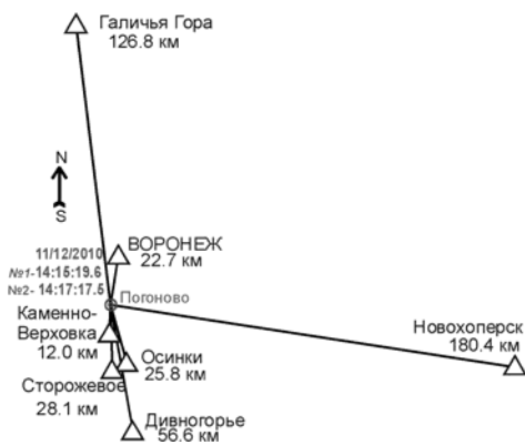
Рисунок 2 – Положение эпицентров взрыва полигона «Погоново» и сейсмических станций локальной и региональной сети
