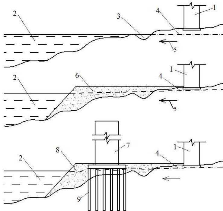
Рисунок 1. Схематический разрез территории: 1- строящийся объект; 2- река; 3- пойменная территория; 4- уровень грунтовых вод; 5- направление разгрузки грунтовых вод; 6- намытая территория; 7- строящийся объект; 8-понижение грунтовых вод; 9- свайное основание.
