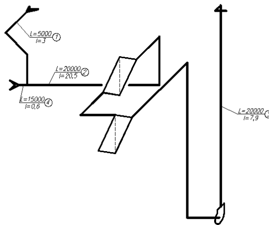
Рисунок 3. Схема аспирационной сети от дробильной установки.
