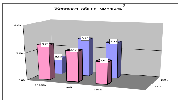
Рисунок 3- Динамика изменения показателя общей жесткости и рН апрель-июнь 2010, 2011 года.
