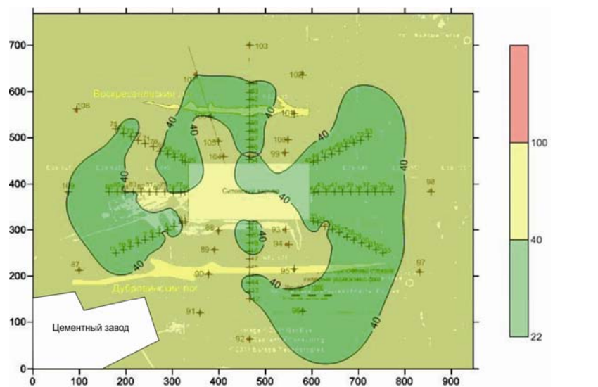
Рисунок - 3 Эколого-геохимическая карта по загрязнению района медью
