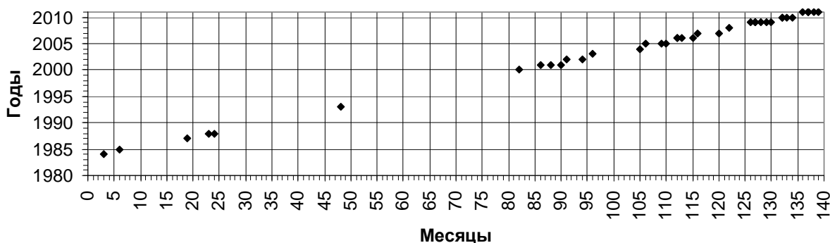
Рисунок 1. Каталог использованных для анализа сцен Landsat по Воронежскому водхр.
