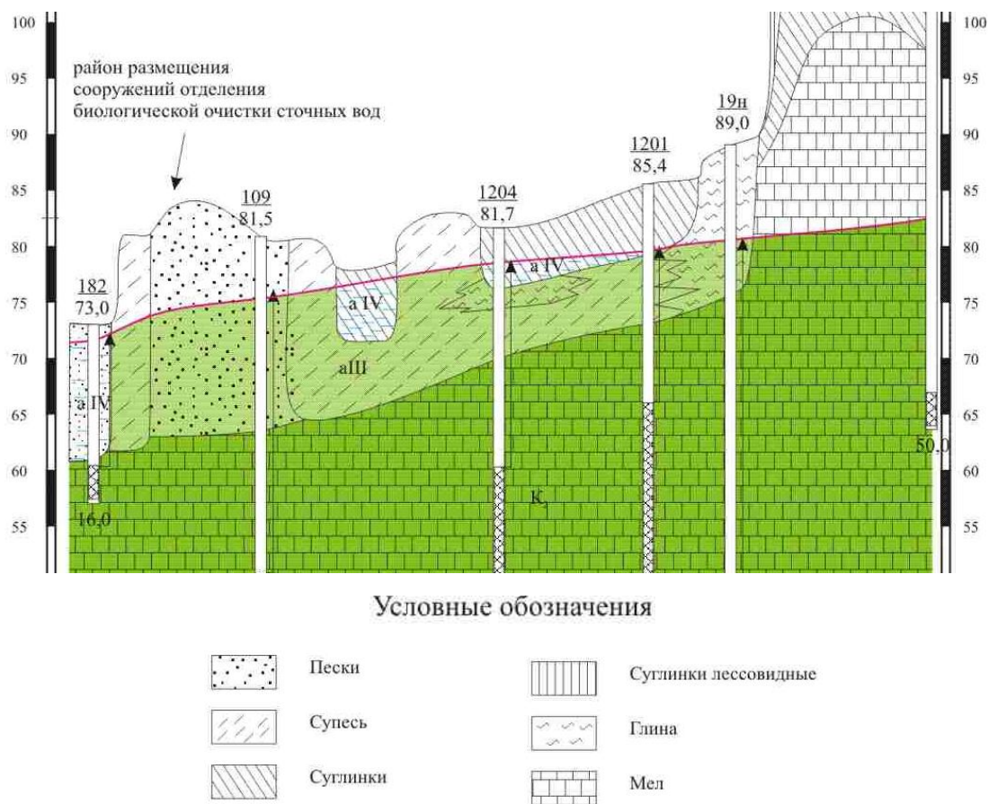
Рис. 4. Схематический гидрогеологический разрез
