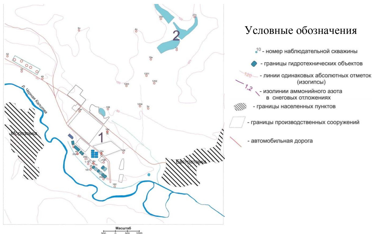
Рис. 3. Схема основных источников загрязнения подземных вод
