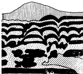
Рис. 12. Нарушение слоистости донных осадков пескожилом. Штриховкой и другими условными обозначениями показаны осадки разного состава (по Алексе-ву и Найдину, 1973)
