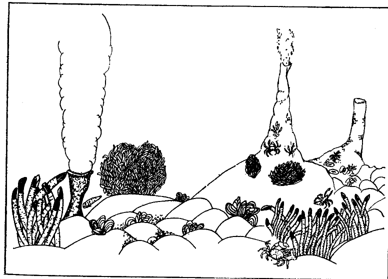
Рис. 3. Абиссальное рифтовое сгущение жизни. На переднем плане — рифтии (слева и справа), двустворчатые моллюски (среди «подушечной лавы»), крабы, рыбы. На среднем и заднем плане — «черные курильщики» (в виде труб) и «белые курильщики», покрытые «зарослями» полихет. На заднем плане справа — прекративший свое существование «черный курильщик» с распавающимся сообществом организмов
