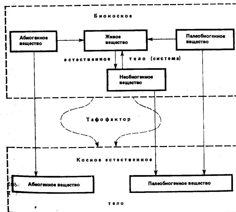
Рис. 9. Схема формирования осадочных пород в биокосных системах с последующим захоронением
