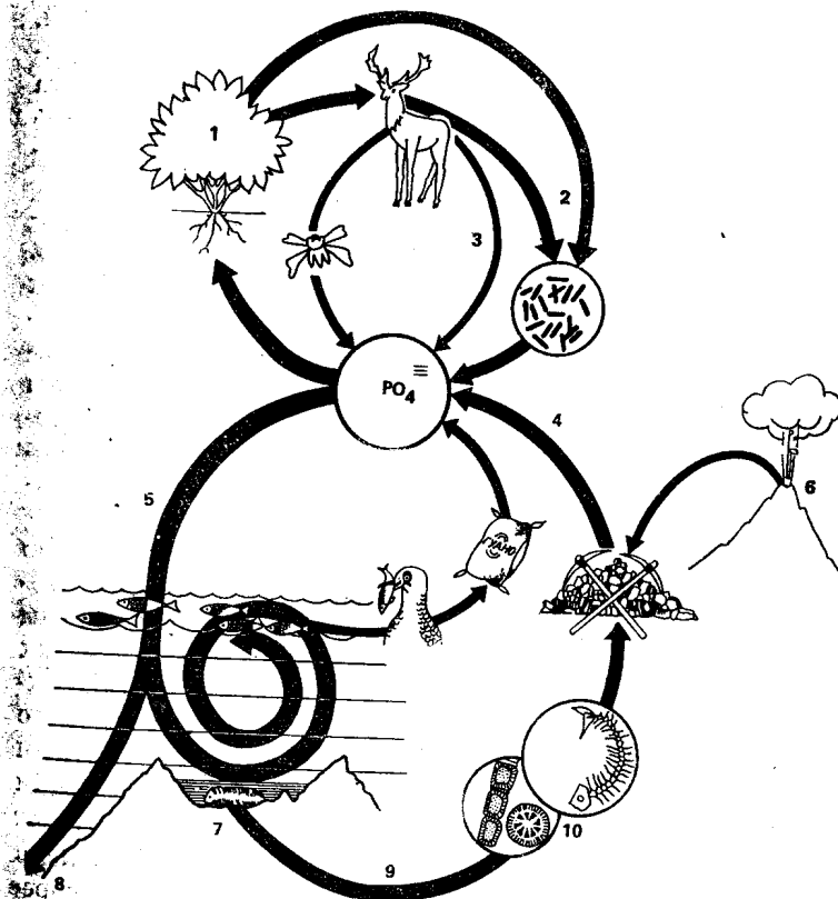
Рис. 15. Схема биогеохимического цикла фосфора (по Дювиньо, 1974): 1 — накопление фосфора высшими растениями; 2 — разложение небиогенного органического вещества; 3 — экскременты; 4 — эрозия; 5 — поступление в океан; 6 — вулканический апатит; 7 — осаднение на небольшой глубине; 8 — осаднение на значительных глубинах; 9 — переход в ископаемое состояние; 10 — включение в биотический круговорот диатомовыми водорослями
