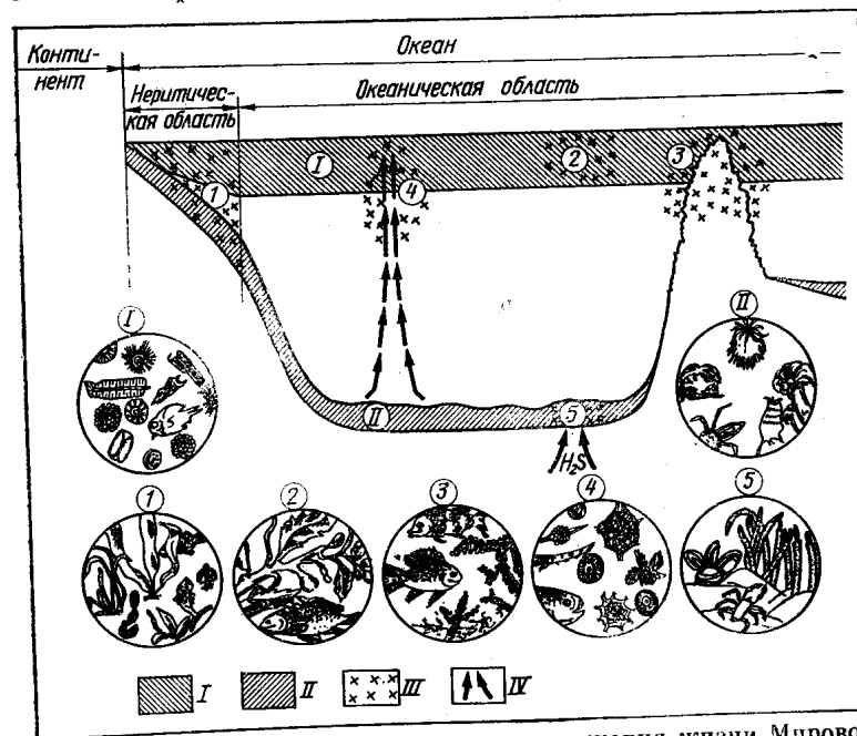
Рис. 2. Экогоризонты, концентрации и разрежения жизни Мирового океана: I — планктонная пленка жизни; II — донная пленка жизни; III — сгущения жизни; I — прибрежное; 2 — саргассовое; 3 — рифовое; 4 — апвеллинговое; 5 — абиссальное рифтовое; IV — разрежение жизни в глубинных водах; A — разрежение жизни
