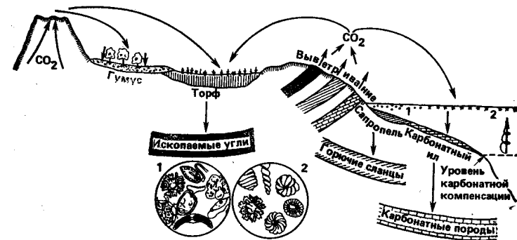
Рис. 14. Схема формирования каустобиолитов и карбонатных пород в биосфере: 1 — организмы — сапропелеобразователи; 2 — карбонатные организмы
