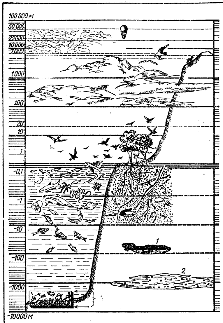
Рис. 1. Распределение живых организмов в биосфере (по Кадару, 1965): 1 — обитатели пещер; 2 — микроорганизмы подземных местобитаний; еще ниже — донная пленка жизни
