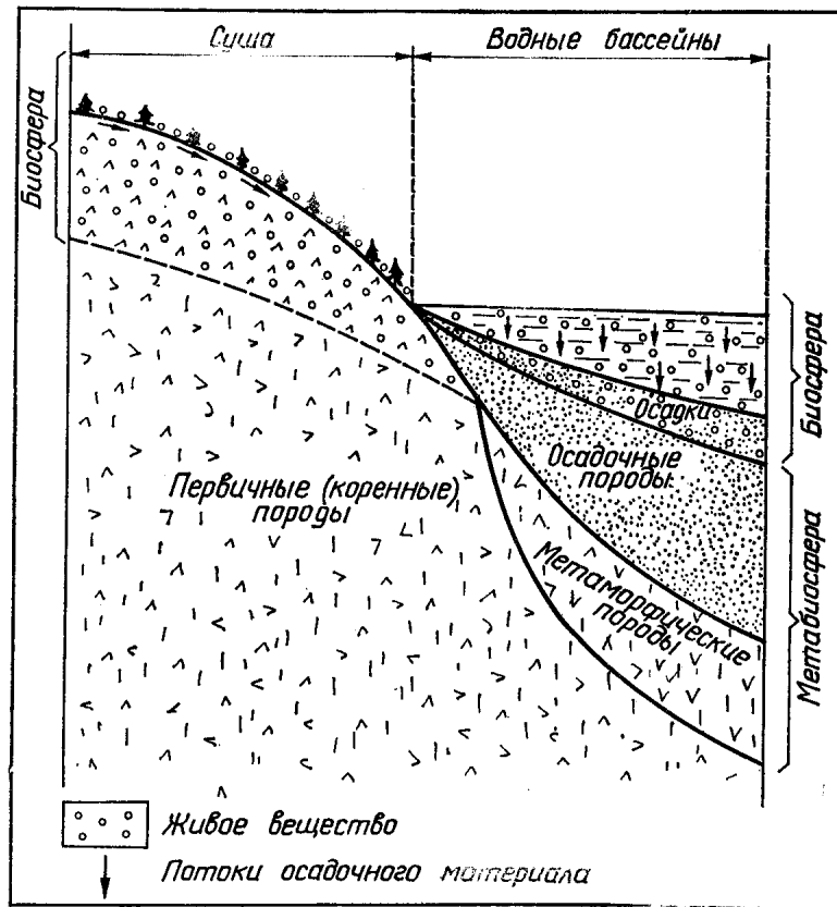
Рис. 10. Схема формирования горных пород метабиосферы
