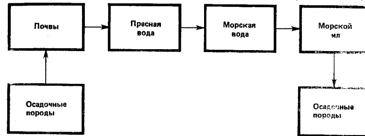
Рис. 7. Принципиальная схема формирования осадочных пород (по Вернадскому, 1936)
