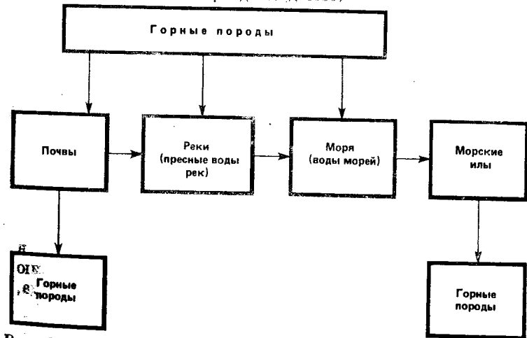
Рис. 8. Принципиальная схема формирования осадочных пород (по Личкову, 1946)
