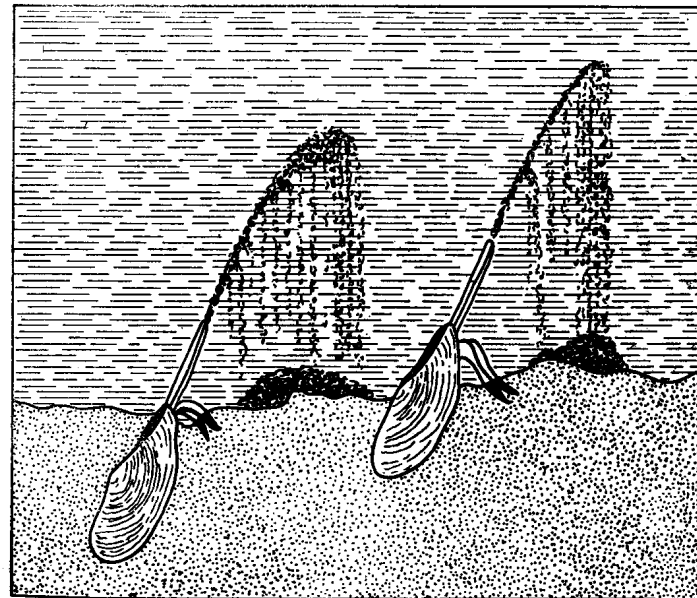
Рис. 11. Переработка донных осадков современным двусторчатым моллюском Ioldia hyperborea (по Йоханссону, 1985)
