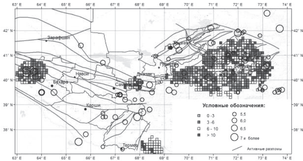
Рис. 5. Площадное распределение нормированной на прочность сцепления величины эффективного давления ( p^*/\tau_f ) для сейсмоактивного слоя, расположенного ниже 15 км
