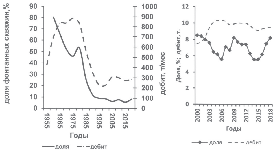
Рис.10. – Доля фонтанных скважин в НГЗ отрасли РФ и среднемесячный дебит. а) по пятилетиям; б) по годам. Этой же теме посвящены также работы [4– 5].
