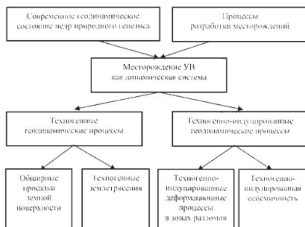
Рис.1. Схема формирования аномальных сейсмических и деформационных последствий разработки месторождений углеводородов (по [Кузьмин, Жуков, 2004]).
