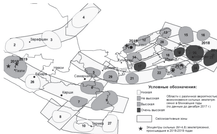
Рис. 3 – Карта областей ожидаемой сейсмической активизации на ближайшие годы по комплексу прогностических параметров сейсмического режима, построенная в 2018 году и переданная МЧС РУз
