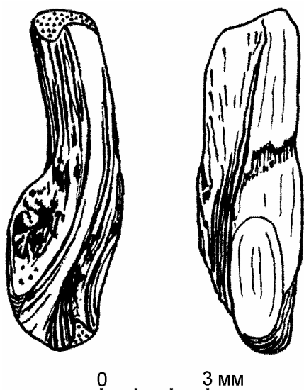
Рис. 1. Кожная сочленовная кость Pliobatrachus cf. langhae сверху и сбоку.
