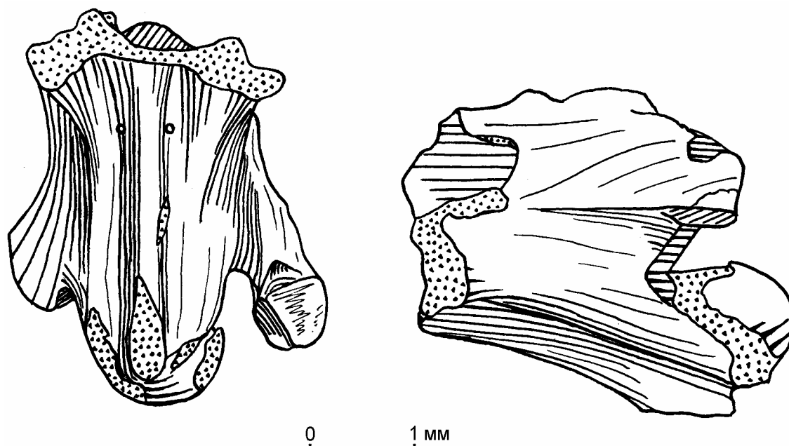
Рис. 4. Туловищный позвонок Vipera sp. снизу и сбоку.
