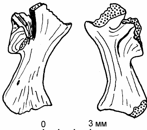
Рис. 2. Лопатка Bufo cf. raddei снаружи и изнутри.
