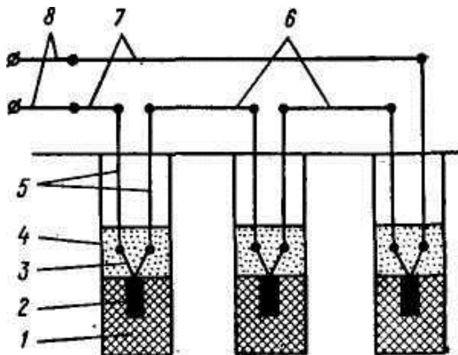
Рис. 23. Схема последовательного соединения электровзрывной сети. 1 — заряд ВВ; 2 — ЭД; 3 — выводной провод электро-детонатора; 4 — забойка; 5, 6, 7, — соединительные провода, 8- магистральные провода.
