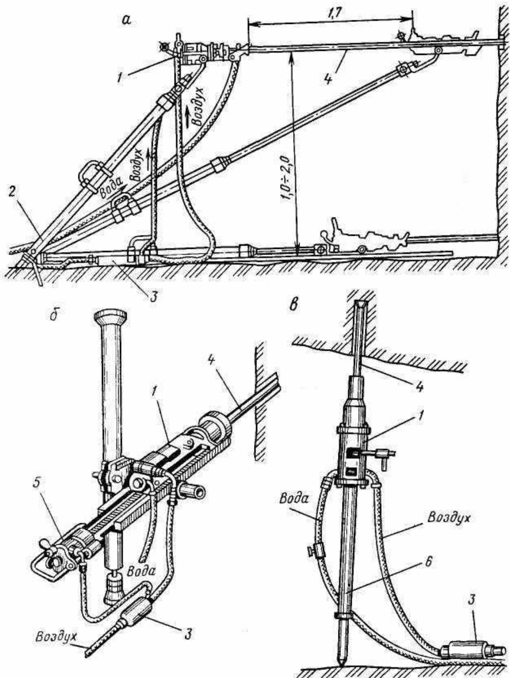
Рис. 8. Типы пневматических перфораторов: а – переносной на пневмоподдержке; б – колонковый; в – телескопный: 1 – перфоратор; 2 – пневмоподдержка; 3 – масленка; 4 – буровая штанга; 5 – автоподагчик; 6 - пневмоподагчик
