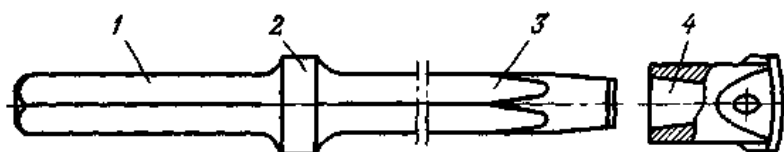
Рис.9. Бур для перфоратора
