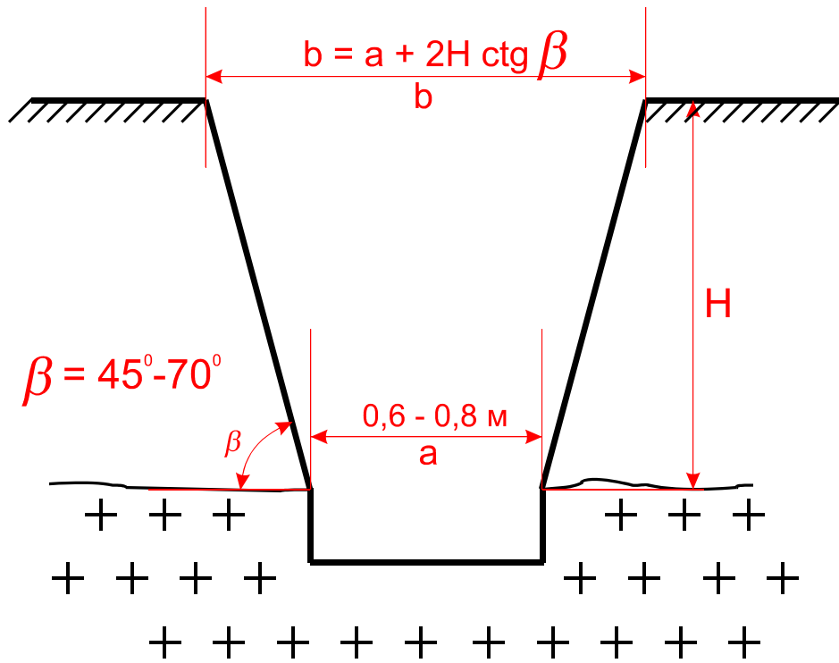
Рис. 1 . Типовое сечение канавы
