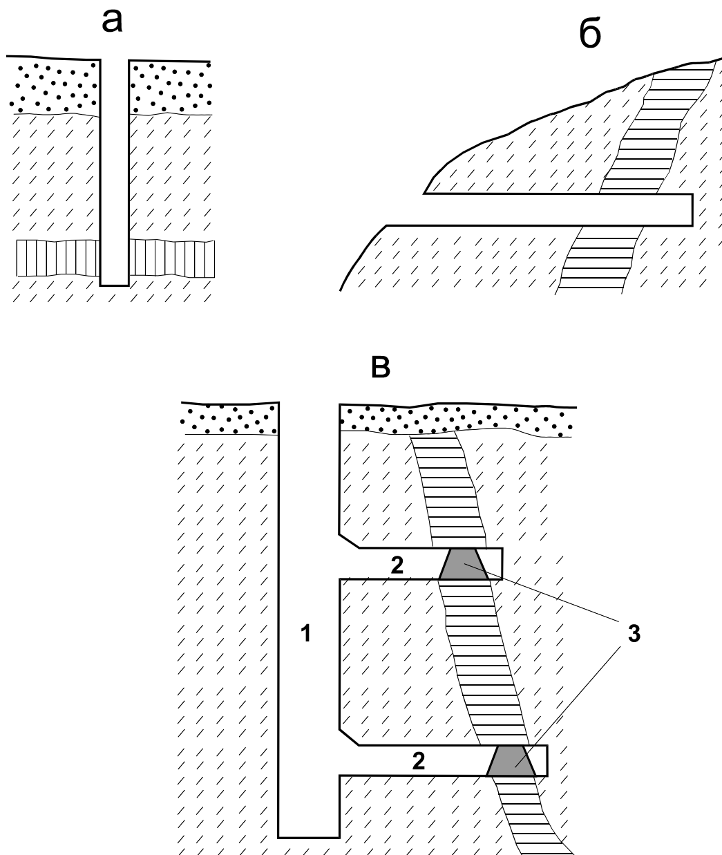
Рис. 4. Подземные горные выработки: а – шурф; б – штольня; в - шахтный ствол (1) с квершлагами (2) и штреками (3).
