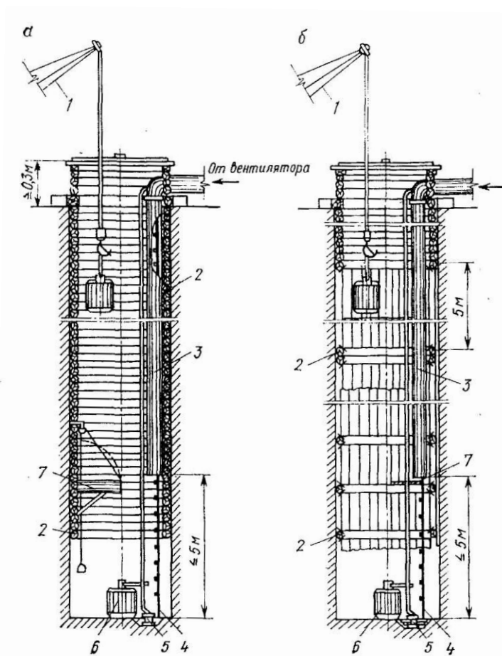
Рис.5.Схема шурфа (проекция на вертикальную плоскость):
