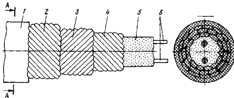
Рис. 19. Детонирующий шнур марки ДШВ: 1, 2, 3 - полихлорвиниловая, хлопчатобумажная и льняная оплетки соответственно; 4 - полиэтиленовая пленка, 5 - взрывчатая смесь из тэна; 6 - направляющие нити.
