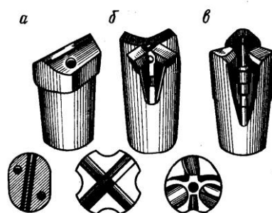
Рис. 10. Типы буровых коронок для перфоратора: а – долотчатая; б – крестовая; в - трехлопастная
