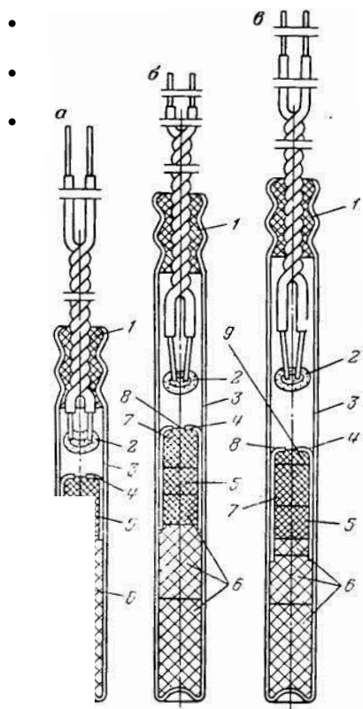
Рис. 21. а, б, в — мгновенного, короткозамедленного и замедленного действия соответственно; 1 — пластиковая пробка; 2 — электровоспламенитель; 3 - гильза детонатора-4 — чашечка; 5, 6 — первичное и вторичное инициирующее ВВ; 7, 9 - замедленный и зажигательный составы; 8-шелковая сетка время замедления 25-250 мс 0,5-10 с.
