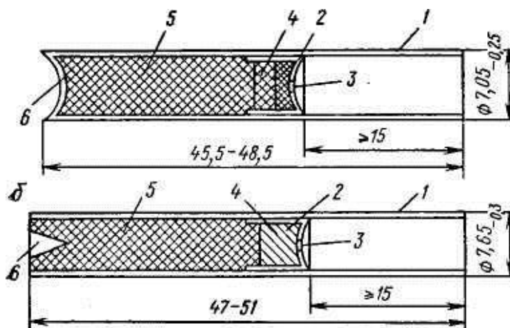
Рис. 20. Капсюль-детонатор: а, б — в металлической и бумажной гильзах; 1 - гильза; 2 - чашечка; 3 - отверстие; 4, 5 - первичный и вторичный инициаторы; 6 - донышко, вогнутое для концентрации энергии взрыва.
