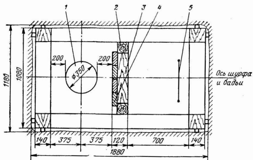
Рис. 6. Типовое прямоугольное сечение шурфа с венцовый крепью:
