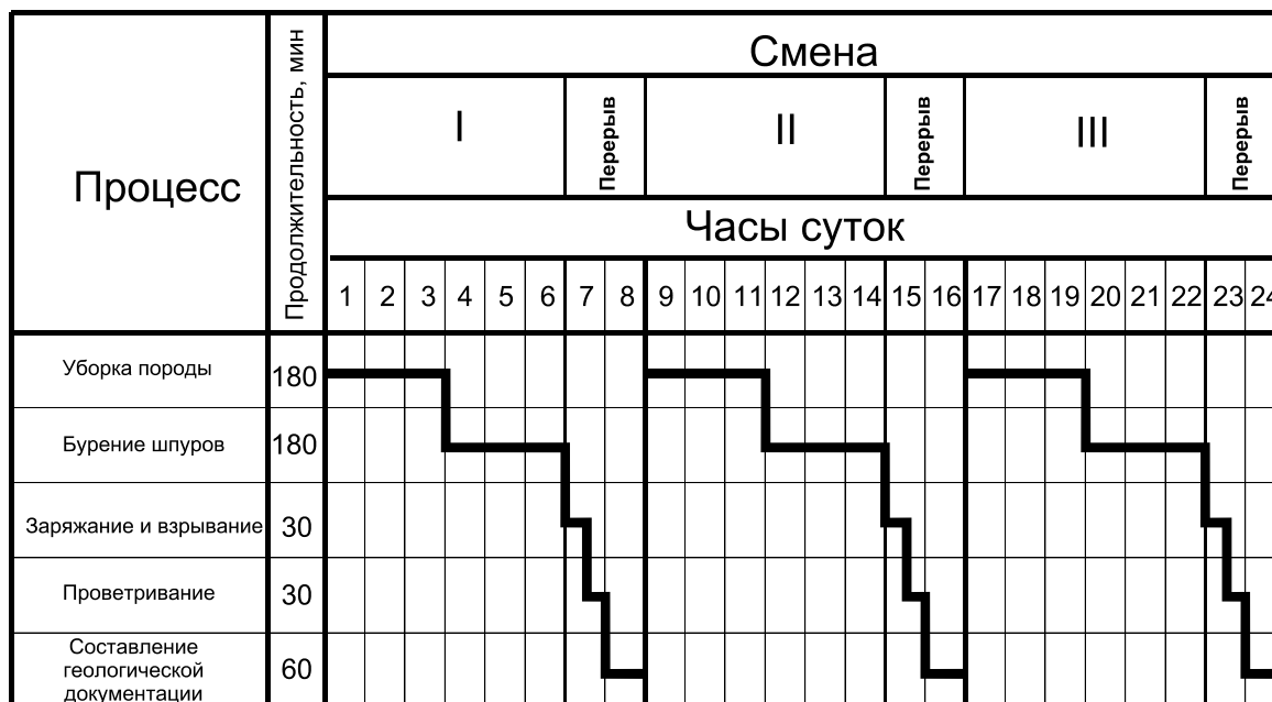
Рис. 7. График циклической организации работ
